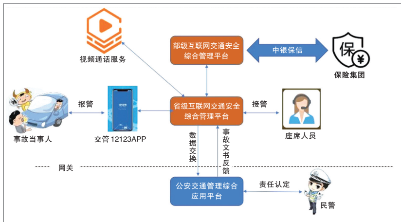
交通事故视频快处系统流程示意图。
