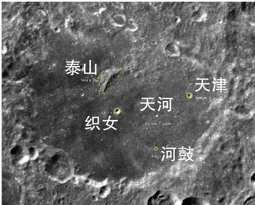
嫦娥四号着陆区地理实体命名影像图。
